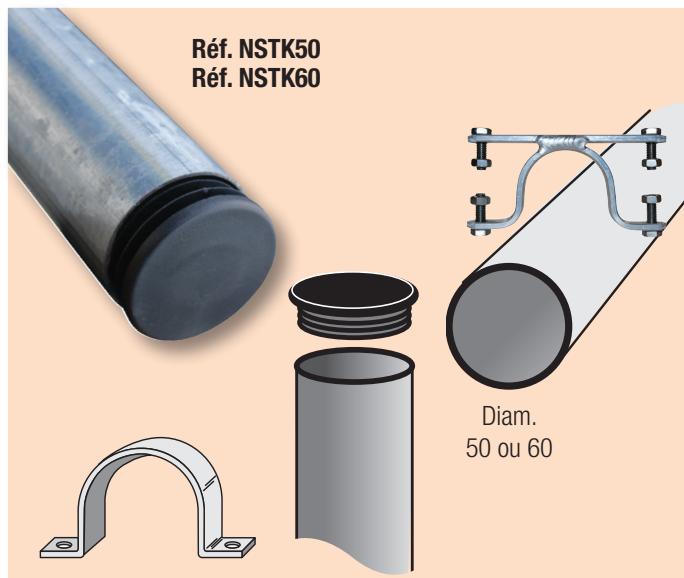
Poteau NSTK60 : Ø 60 mm
