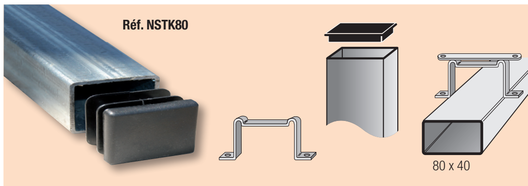
Poteau NSTK80 : 80 x 40 mm
