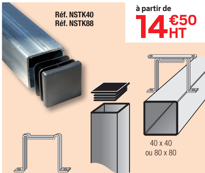
Poteau NSTK40 : 40 x 40 mm
